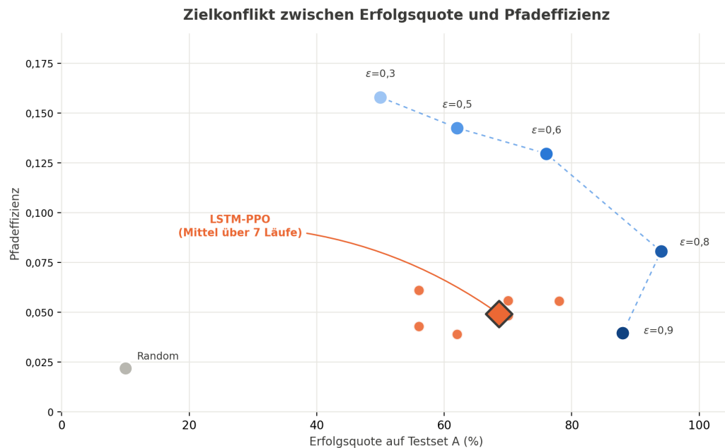
Abbildung 5.5: Evaluation – Erfolgsquote gegen Pfadeffizienz für alle Verfahren, eigene Darstellung.
